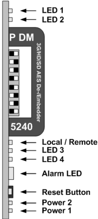
Figure 4: Card Edge
